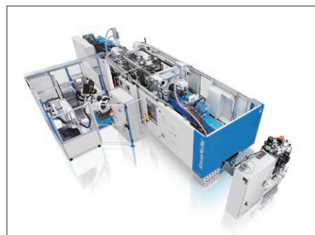
型内塗装：自動車の塗装工程において、金型内で樹脂成形と表面塗装を一工程で行う技術
